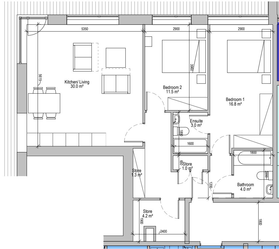
① AT12 83.7 SQM 1 : 100
